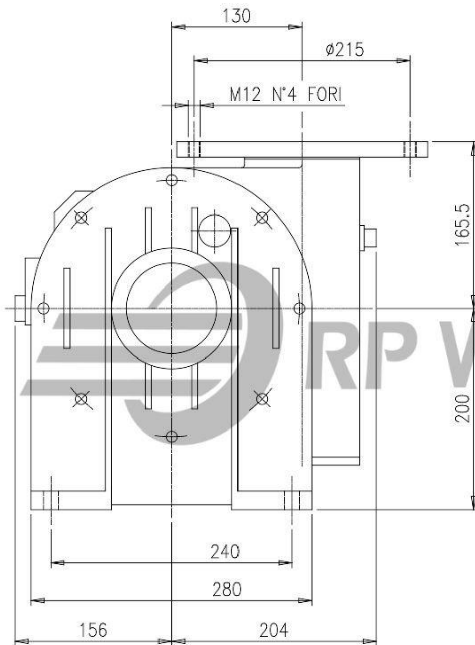
MI 130 V PAM 100 B5
